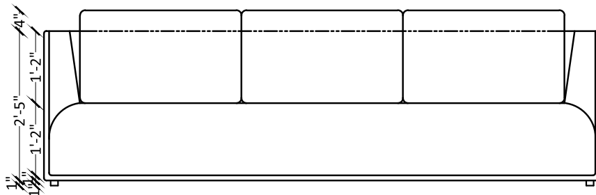
ELEVATION
