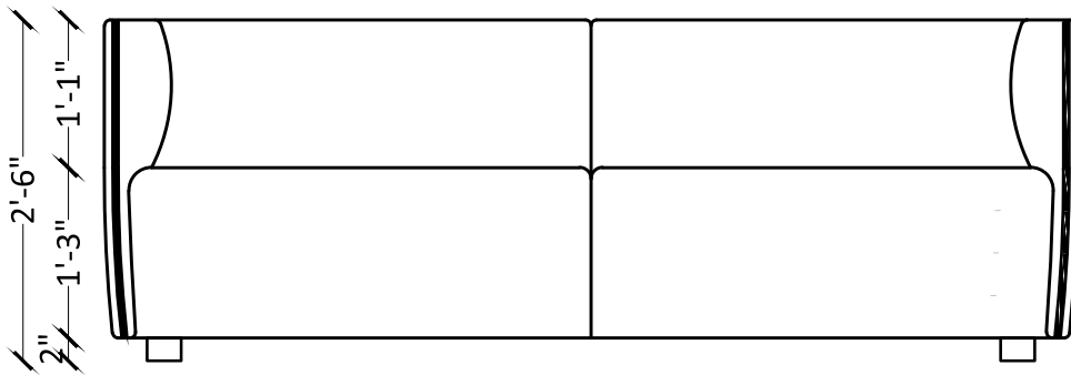
ELEVATION
